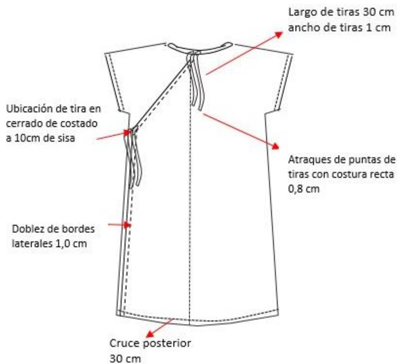
GRÁFICO 2: DESCRIPCIÓN DE COSTURAS ESPALDA
